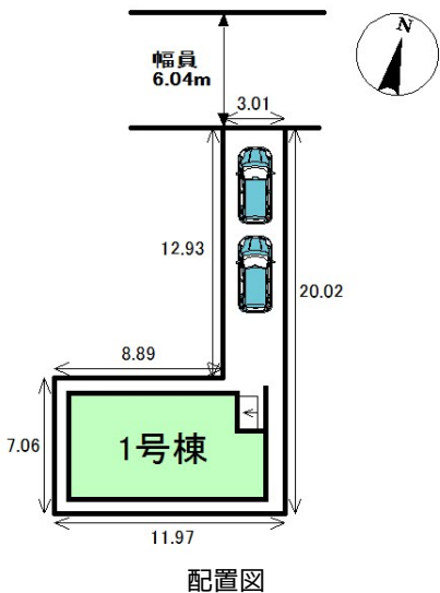
配置図
