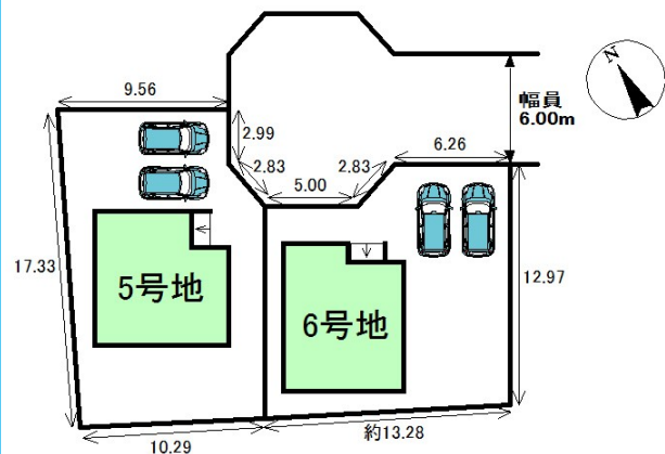
配置図
