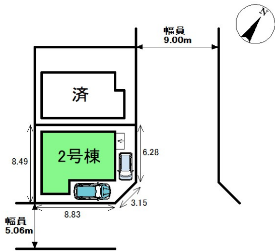
配置図
