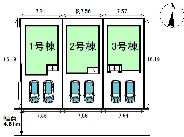
配置図
