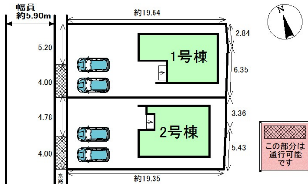
配置図
