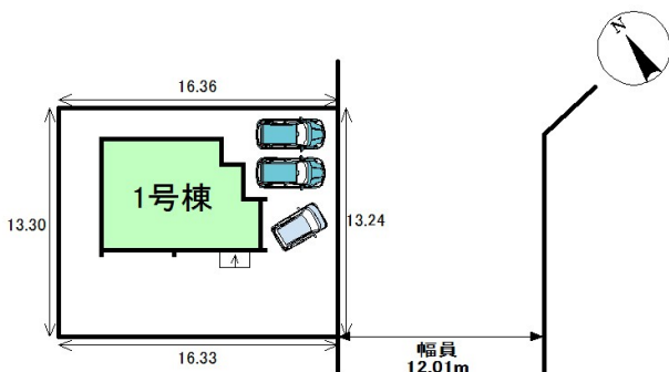
配置図
