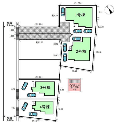
配置図
