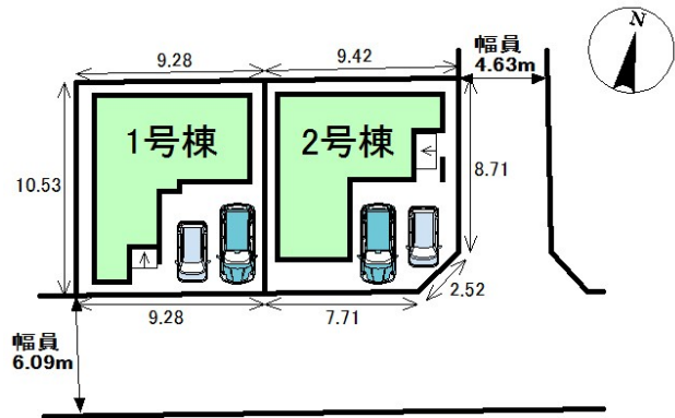
配置図
