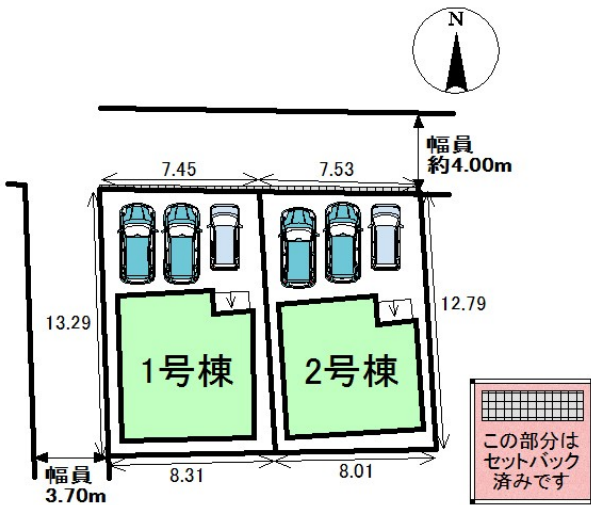
配置図
