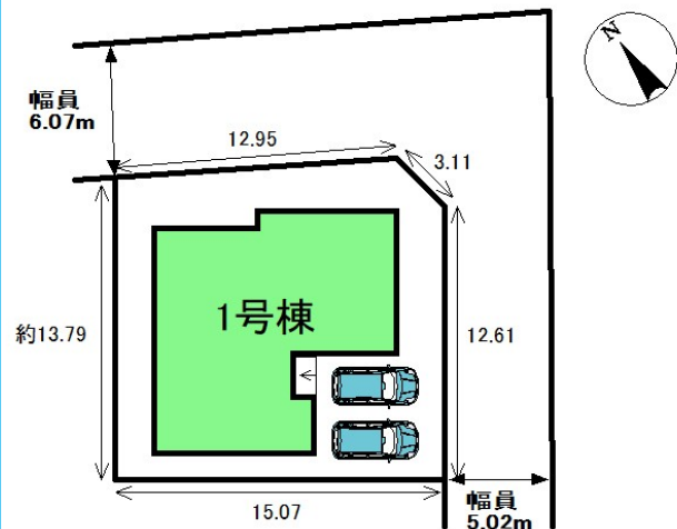
配置図
