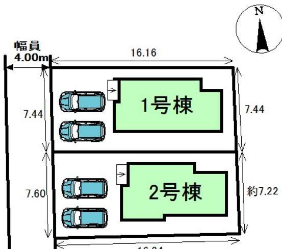
配置図
