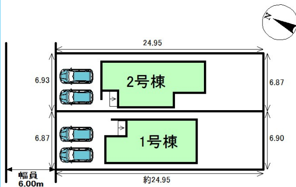
配置図
