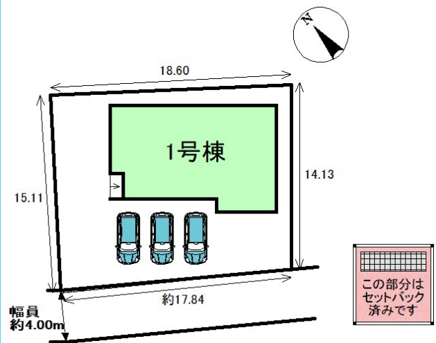
配置図
