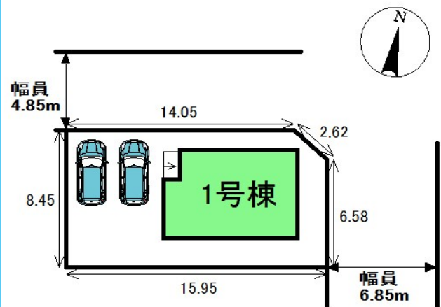
配置図
