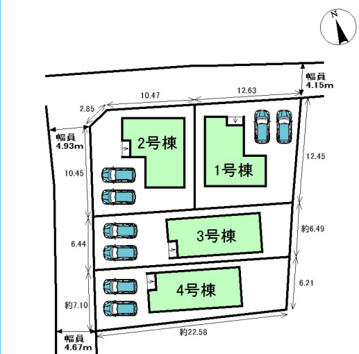
配置図
