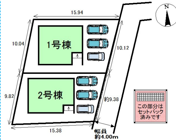
配置図
