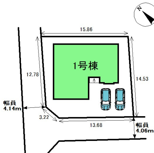
配置図
