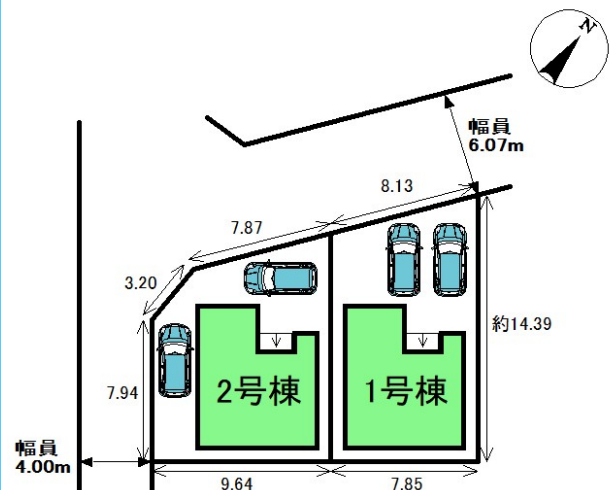
配置図
