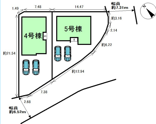
配置図
