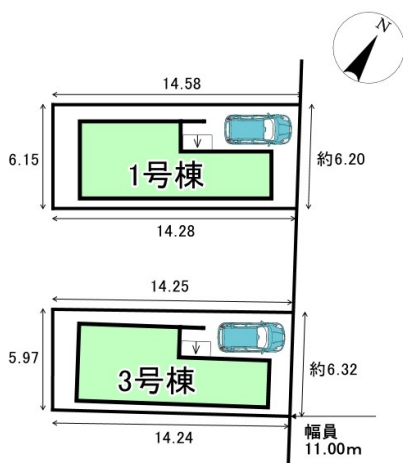
配置図
