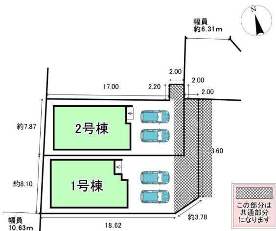
配置図
