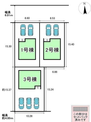
配置図
