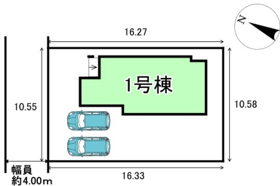
配置図
