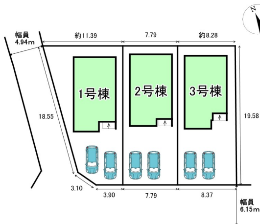
配置図
